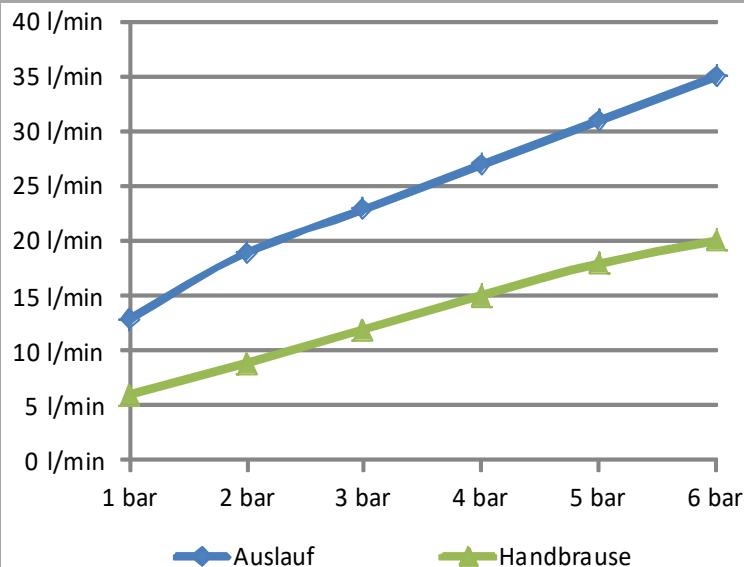
2-Stufige Eco-Kartusche mit Wassersparfunktion
